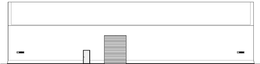
FASAD SL A PORT 3.4x4.5 m, GÅNGDÖRR 1 x 2.1 m
