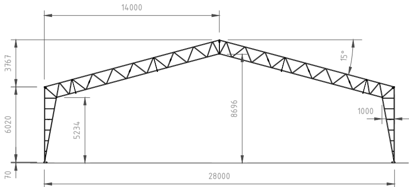
SEKTION SL 2 - 11
