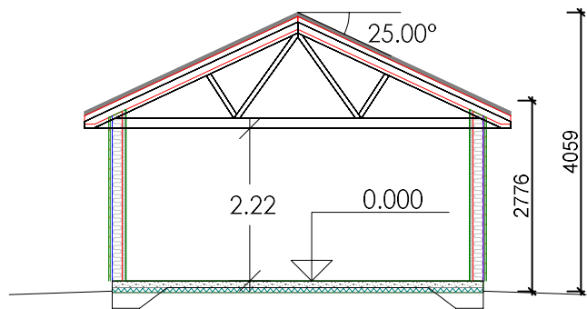
Sektion snitt A-A
