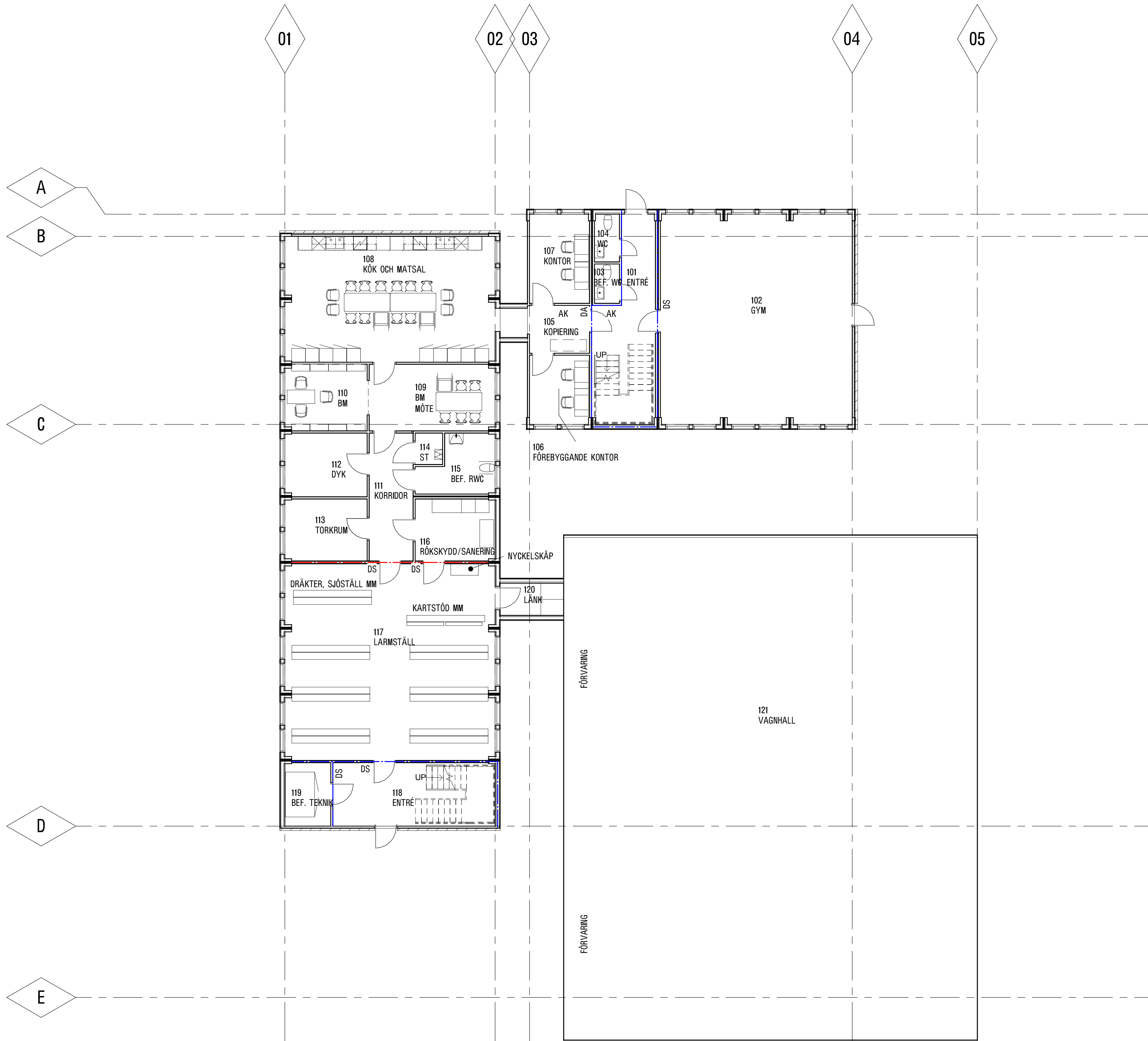
PLAN 1 SKALA 1 : 100
