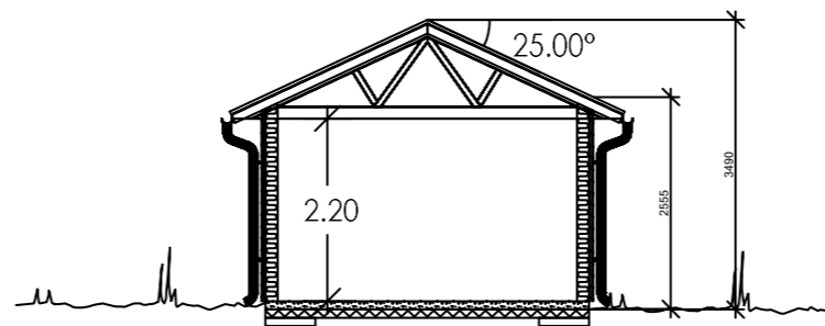
Sektion snitt A-A
