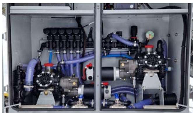
Högtrycks- och högflödesmembranpumpar, motorer och ventiler i slutet kabinett
