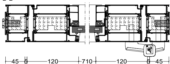
B-B
