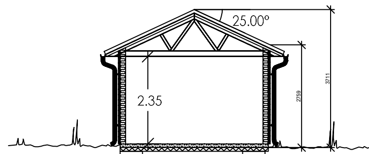
Sektion snitt A-A
